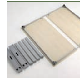
estructura dual classic, patas y canaleta de servicios structure dual classic, pieds et électrification dual classic structure, legs and cable management
