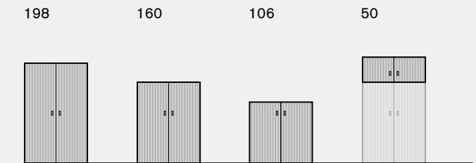
Armarios de lamas / Armoires à rideaux / Tambour cabinets
